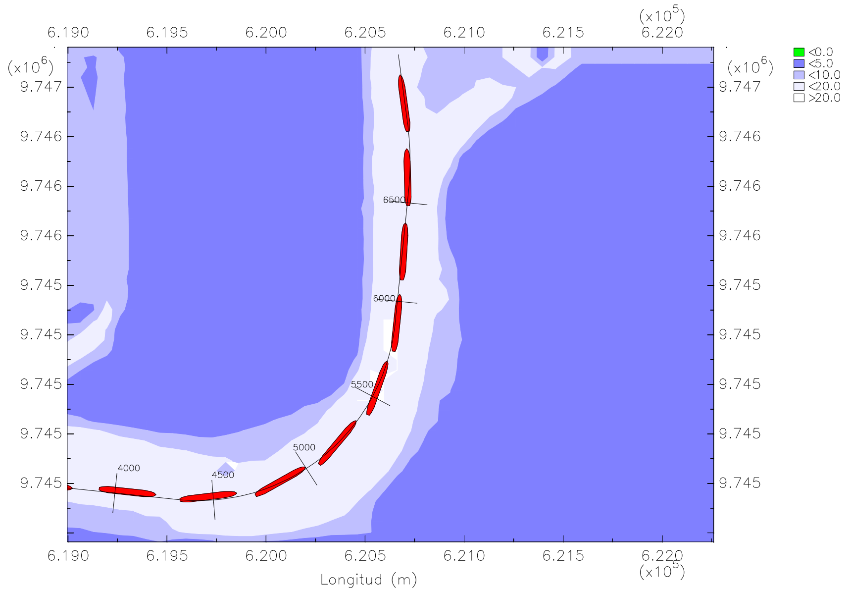
Z3T2 Trayectoria del buque de portacontenedores panamax en flujo
