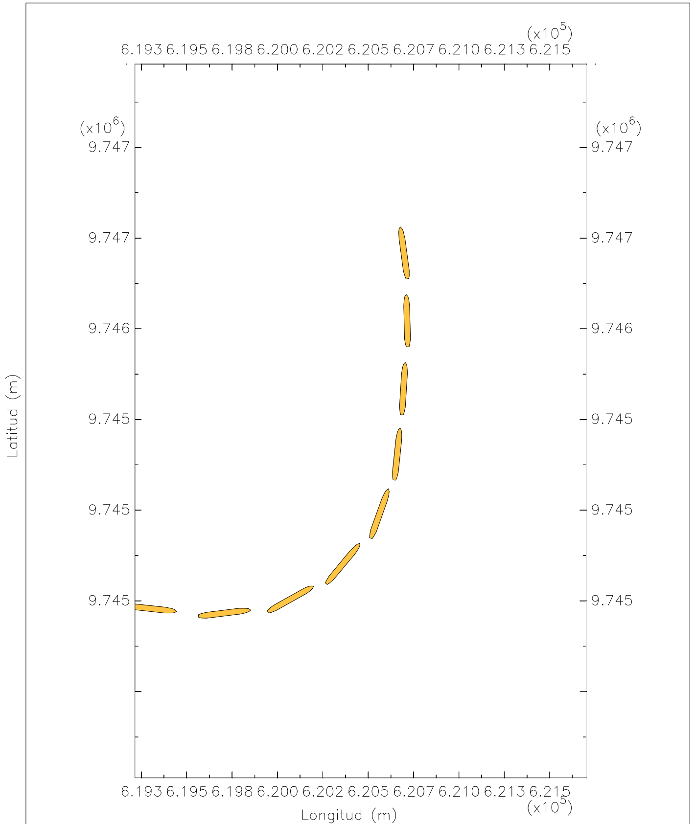
Z3T2 Trayectoria del barco de portacontenedores panamax
